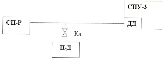
Рисунок 1 – Схема подключения СИ при определении относительной погрешности установок при измерении давления
